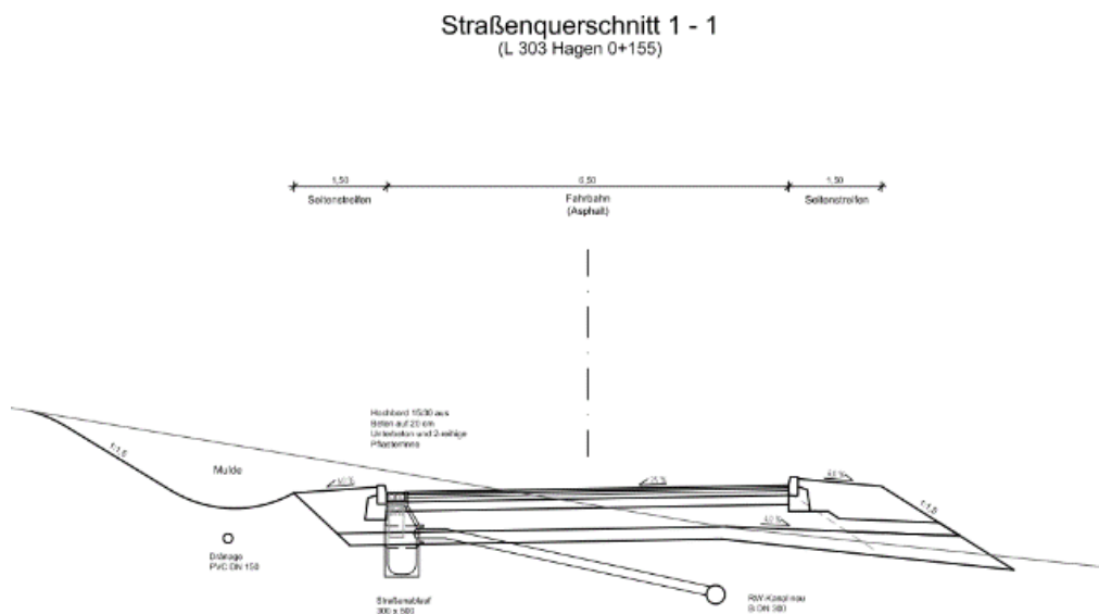
Abb. 2: Straßenquerschnitt 4
